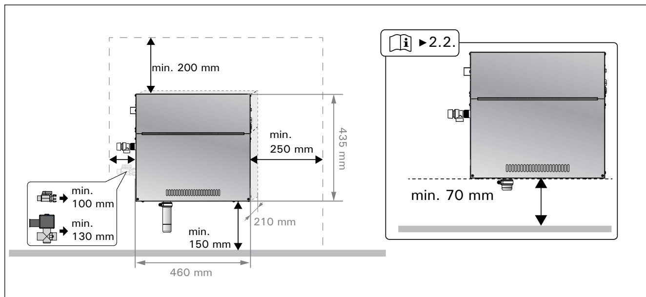
Рисунок 4. Параметры установки Joonis 4. Paigaldusmõõtmed
