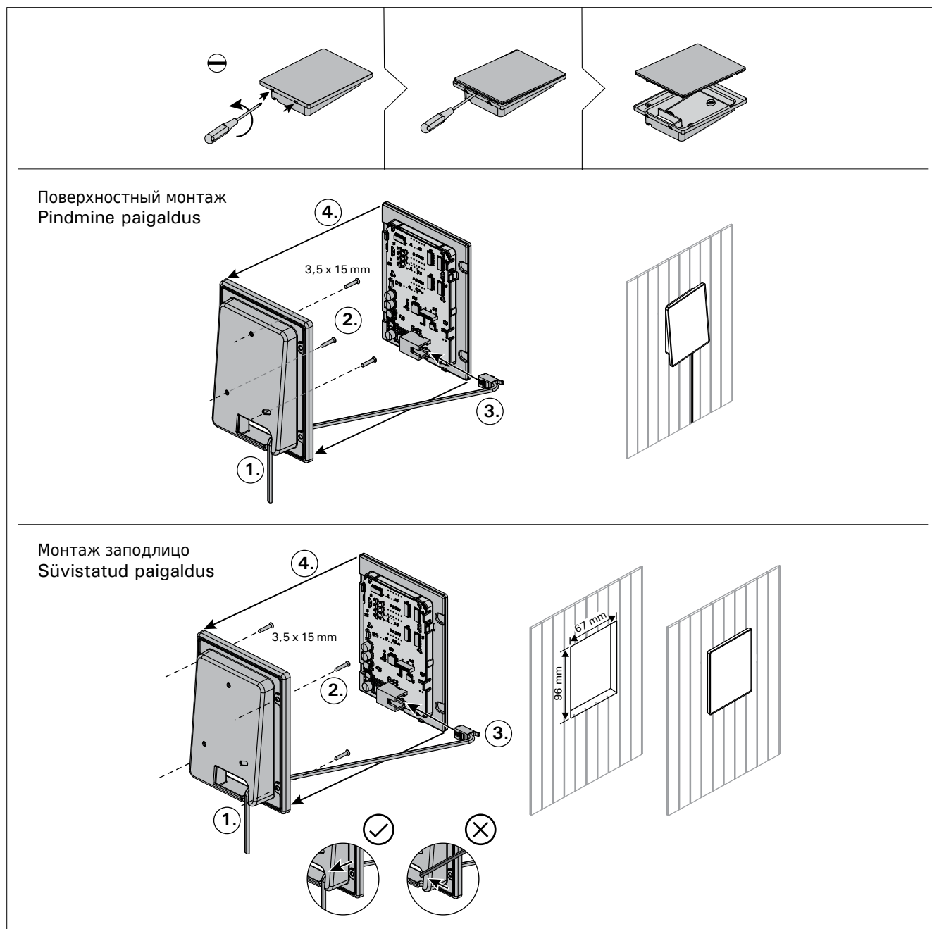
Рисунок 8. Установка панели управления Joonis 8. Juhtpaneeli kinnitamine
