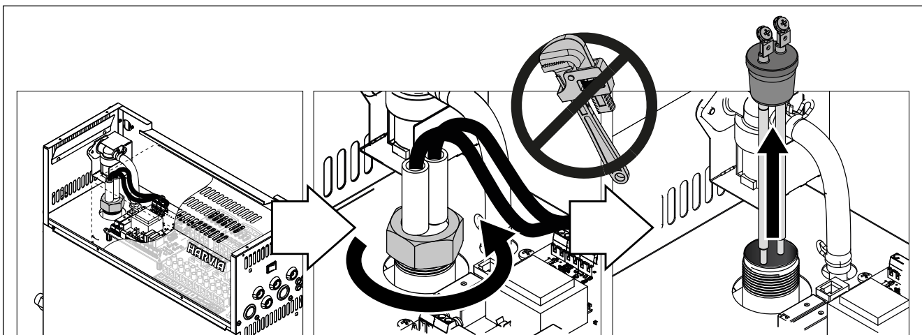
Czyszczenie czujnika poziomu wody Čištění snímače hladiny vody
