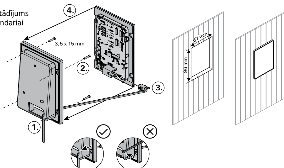
8. zīmējums. Vadības paneļa piestiprināšana 8 pav. Valdymo pults instalavimas
