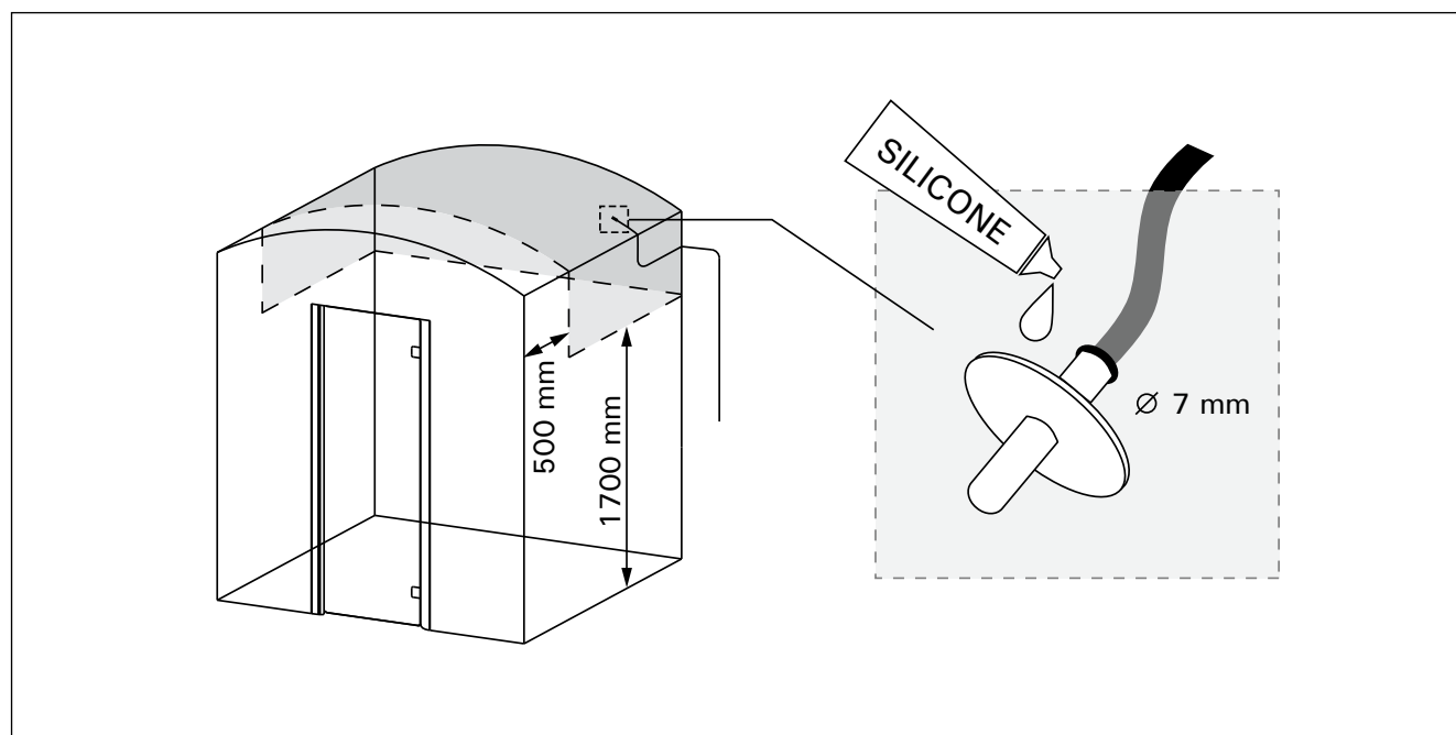
Rysunek 5. Lokalizacja czujnika temperatury Obrázek 5. Umístění teplotního čidla
