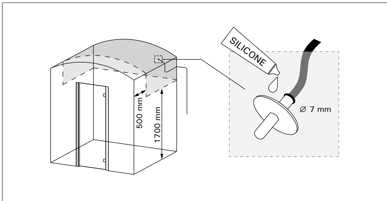
5. zīmējums. Temperatūras sensora ievietošana 5 pav. Temperatūros jutiklio instaliavimas
